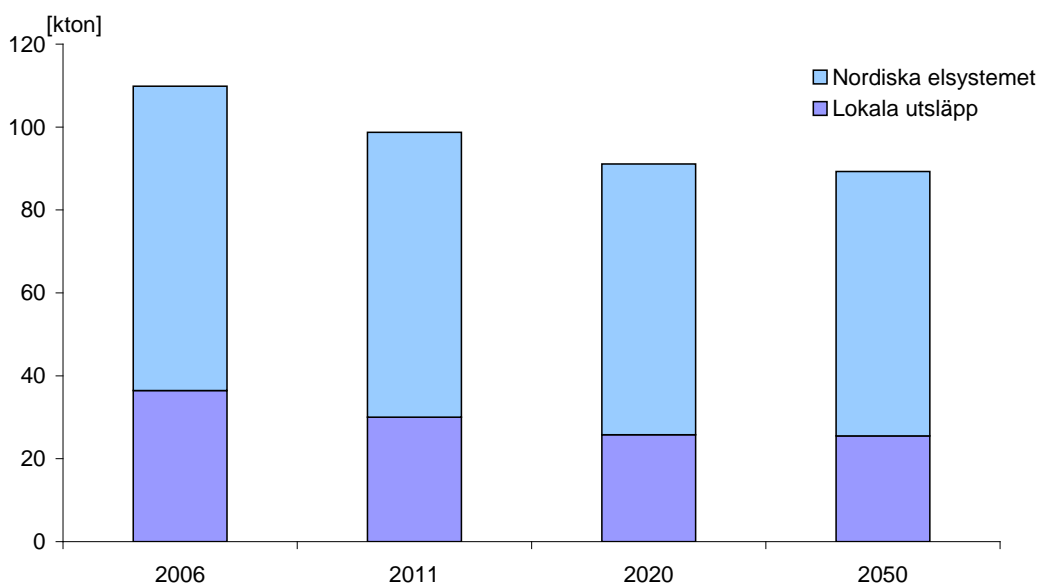
Figur 5: Totala lokala utsläpp av fossilt koldioxid, inklusive utsläppen från fjärrvärme, transporter och industri.
