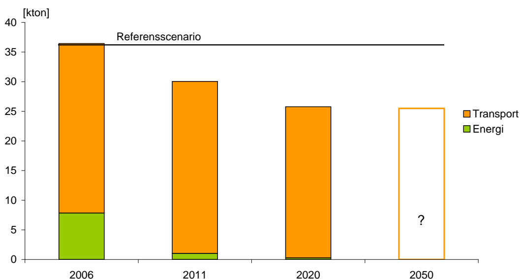
Figur 4: Lokala utsläpp av fossilt koldioxid, inklusive utsläppen från fjärrvärmeproduktion, transporter och industri, exklusive metan och lustgas. Referensscenariot innebär att endast ett fåtal åtgärder genomförs och då ökar utsläppen.
